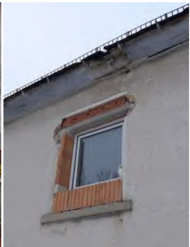
14 b Fassadenmängel, schadhafter Dachrand
