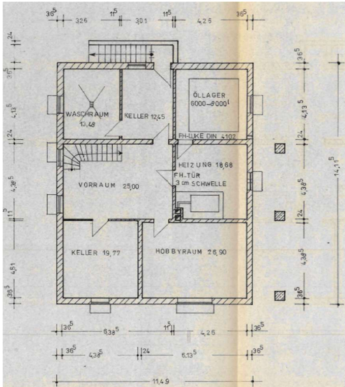
Grundriss Kellergeschoss (ohne Maßstab)
