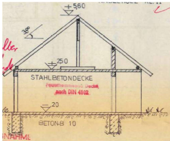
Schnitt B-B (ohne Maßstab)
