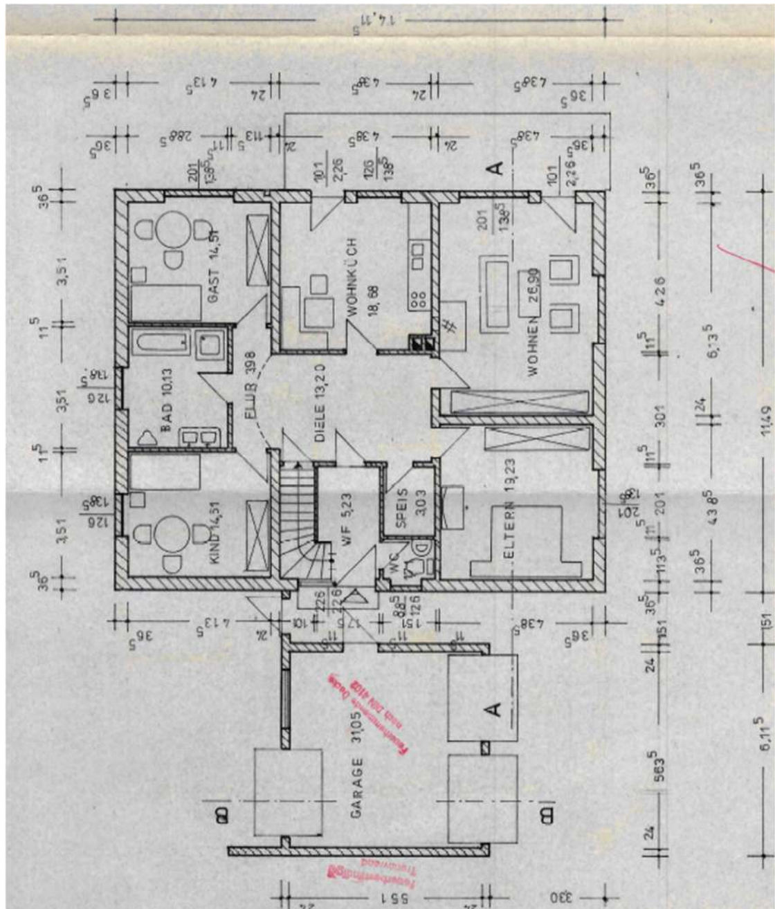
Grundriss Erdgeschoss (ohne Maßstab)
