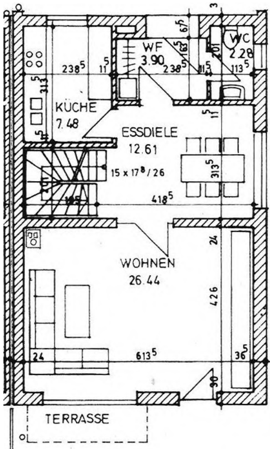
Grundriss Erdgeschoß
