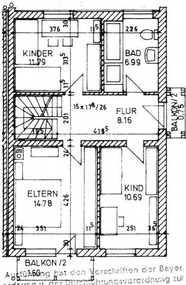
Grundriss Obergeschoß
