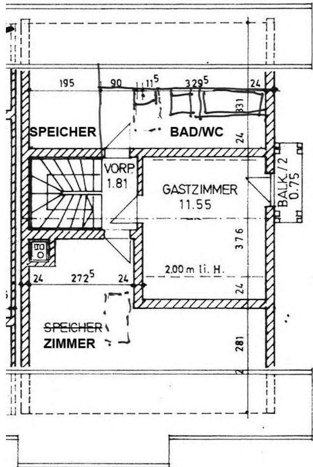
Grundriss Dachgeschoß
