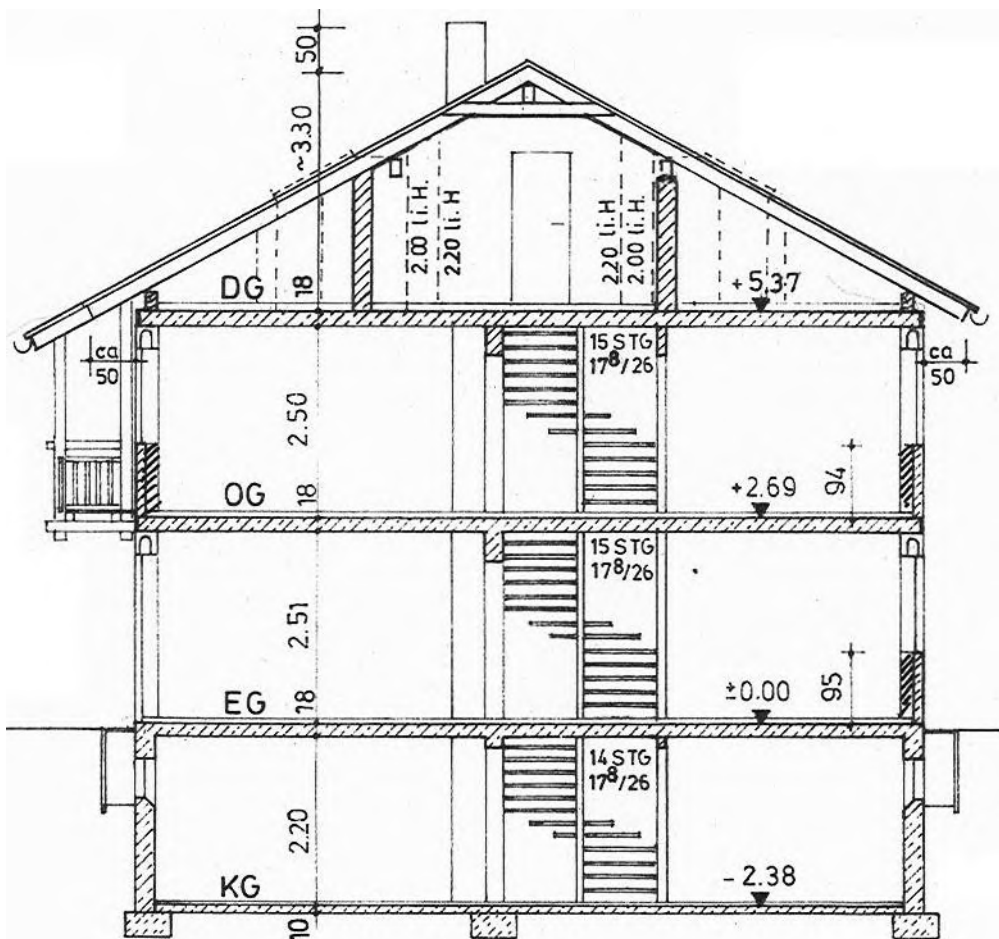
Schnitt
