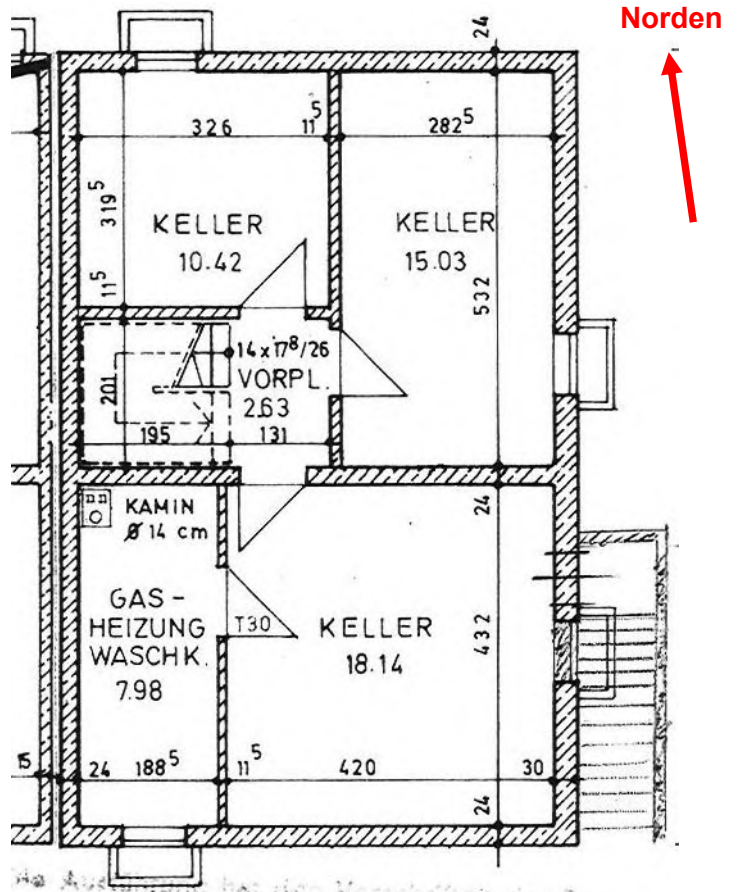
Grundriss Kellergeschoß
