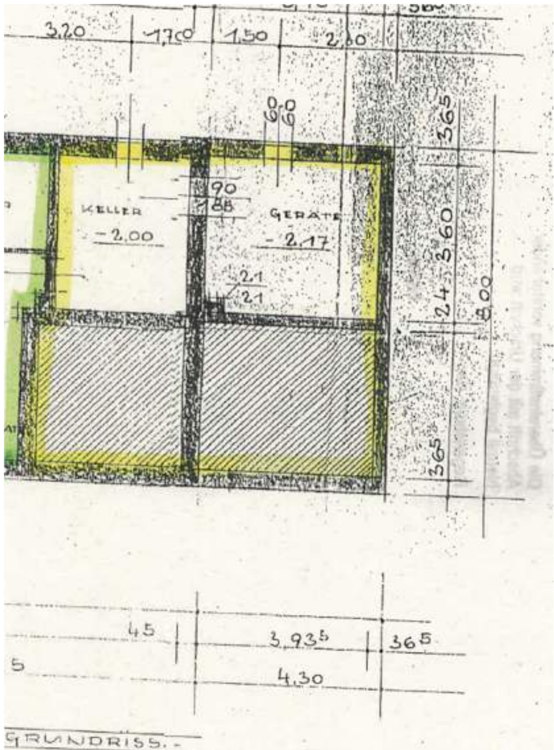
Grundriss Kellergeschoss (ohne Maßstab – Teilbereich nicht auf Grundstück)
