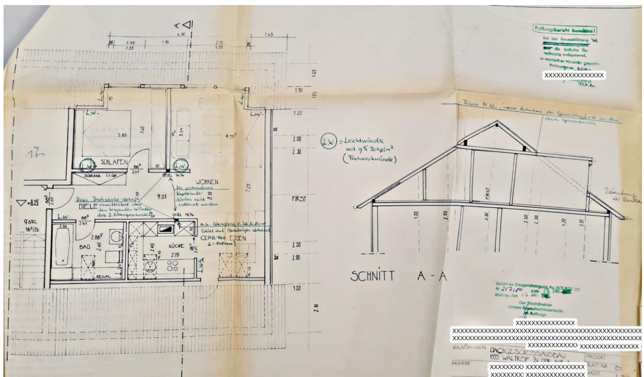
Dachgeschoss rechts
