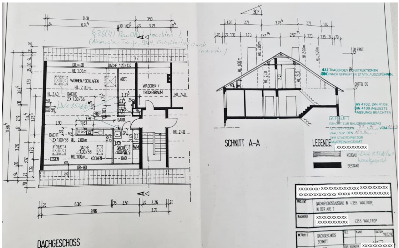
Dachgeschoss links
