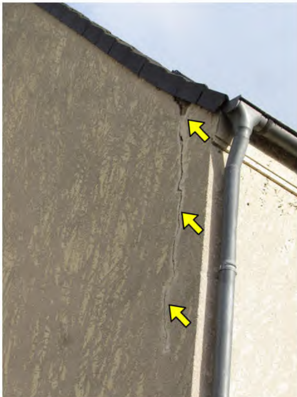
Foto 6: Wohnhaus: Risse in der Giebelwand
