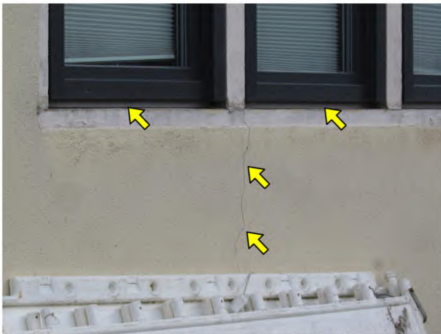
Foto 4: Wohnhaus: Risse in der Fassade, fehlende Außenfensterbänke
