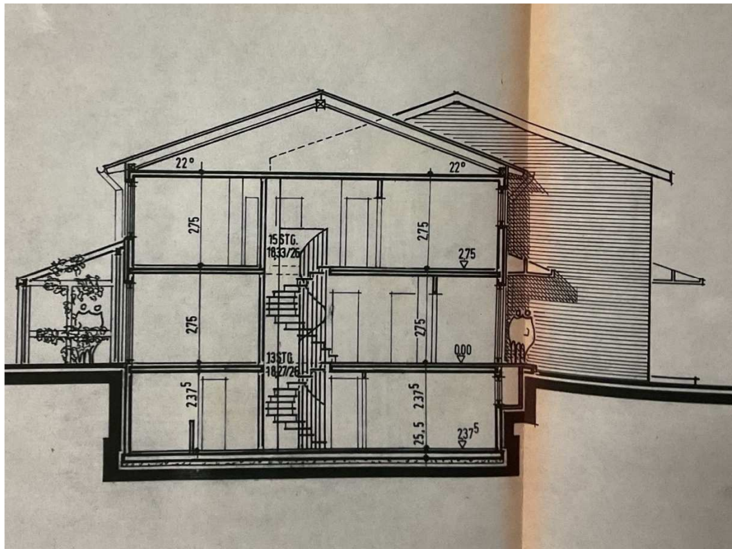
Zeichnung 4: Gebäudeschnitt
