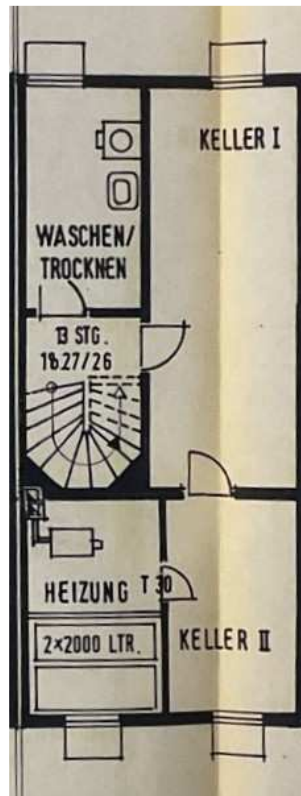
Zeichnung 1: Grundriss Kellergeschoss
