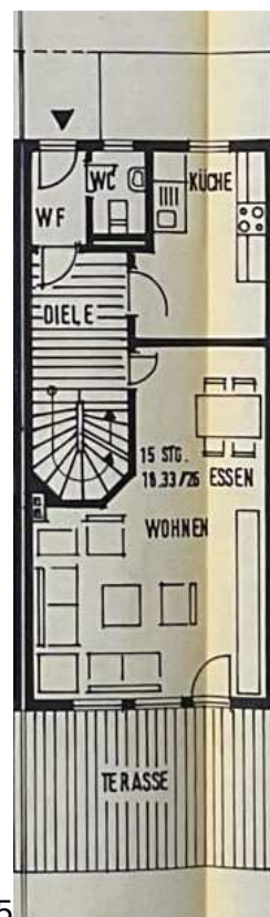
Zeichnung 2: Grundriss Erdgeschoss
