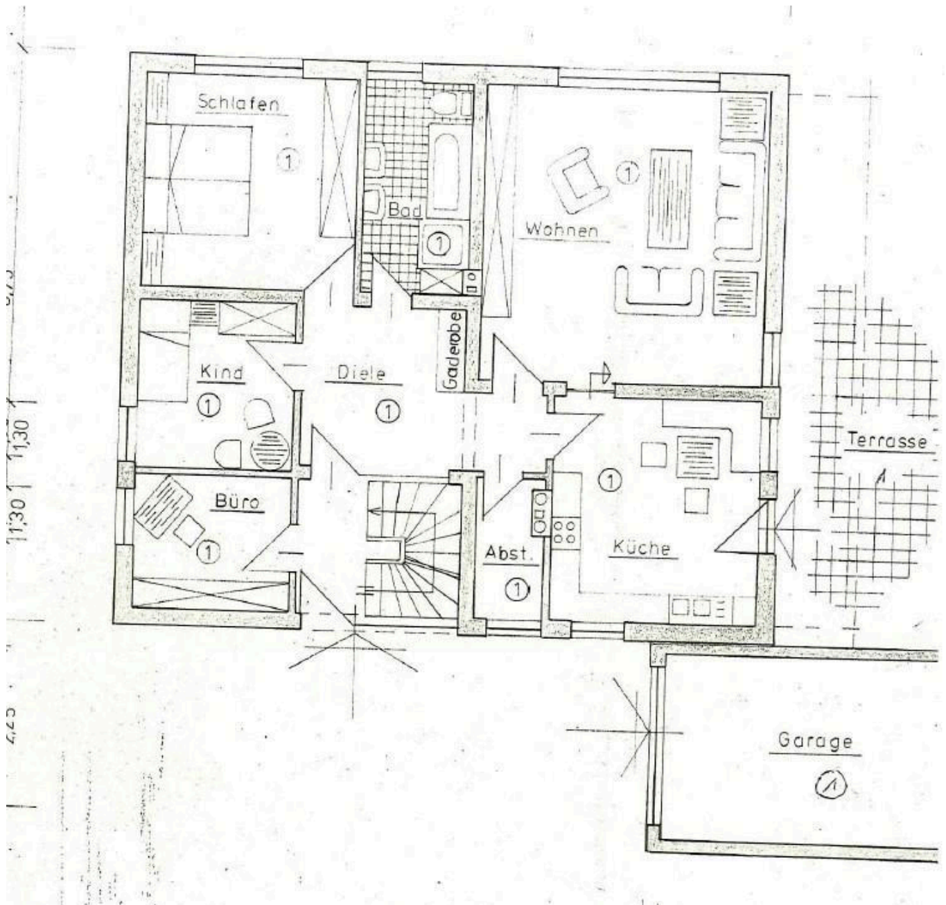
Erdgeschoss WE Nr. 1
