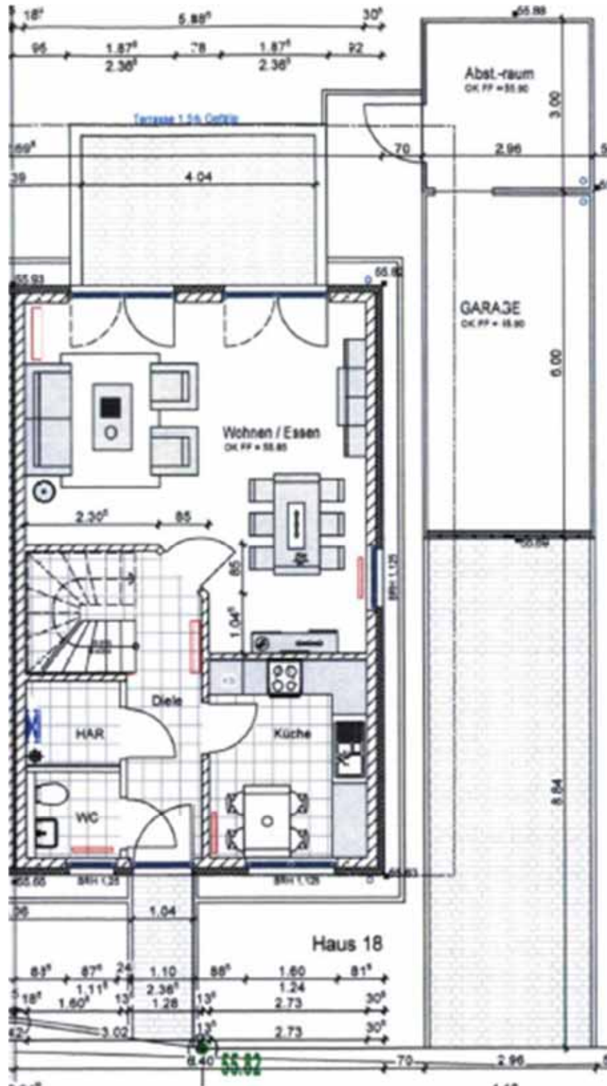
Erdgeschoss
