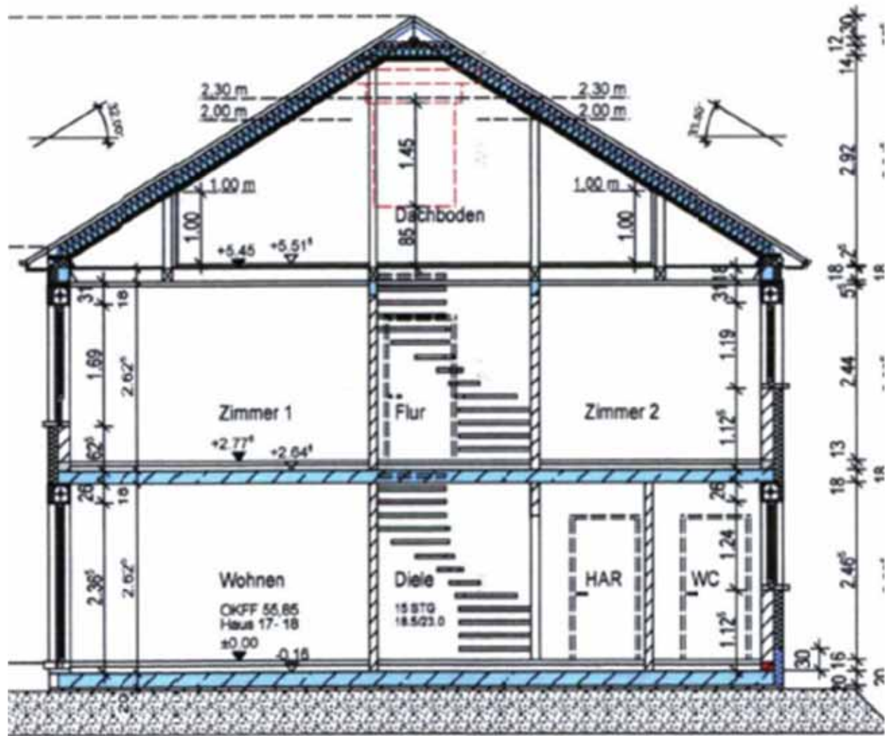
Schnitt A
