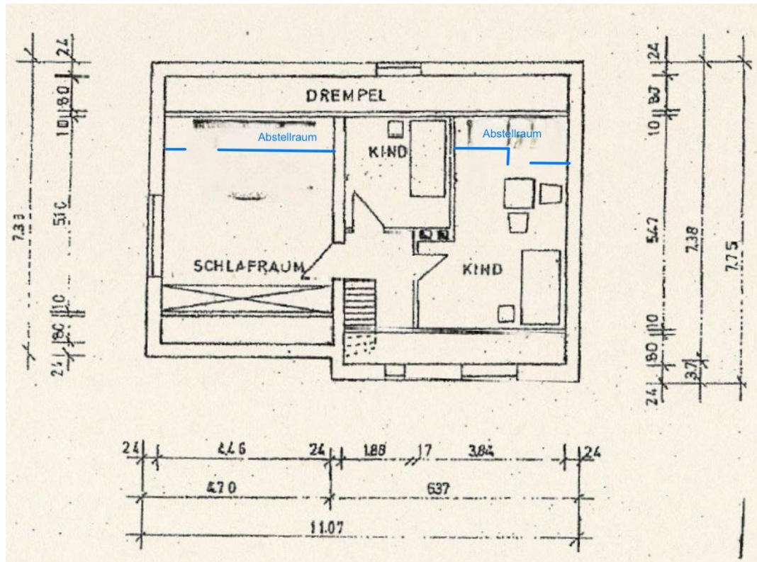
Zeichnung 3: Grundriss Dachgeschoss
