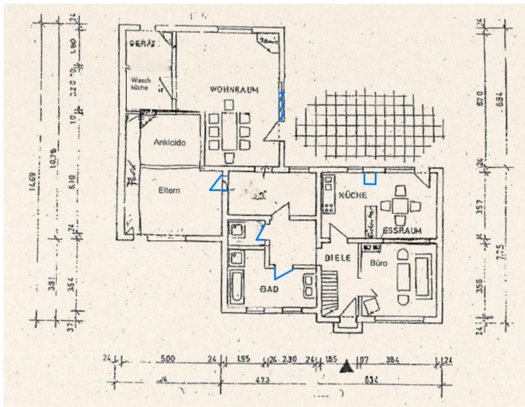
Zeichnung 2: Grundriss Erdgeschoss
