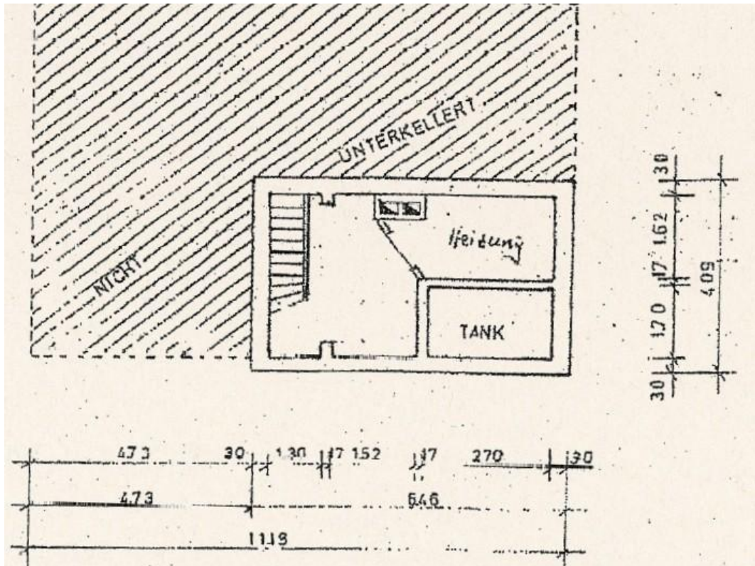
Zeichnung 1: Grundriss Kellergeschoss
