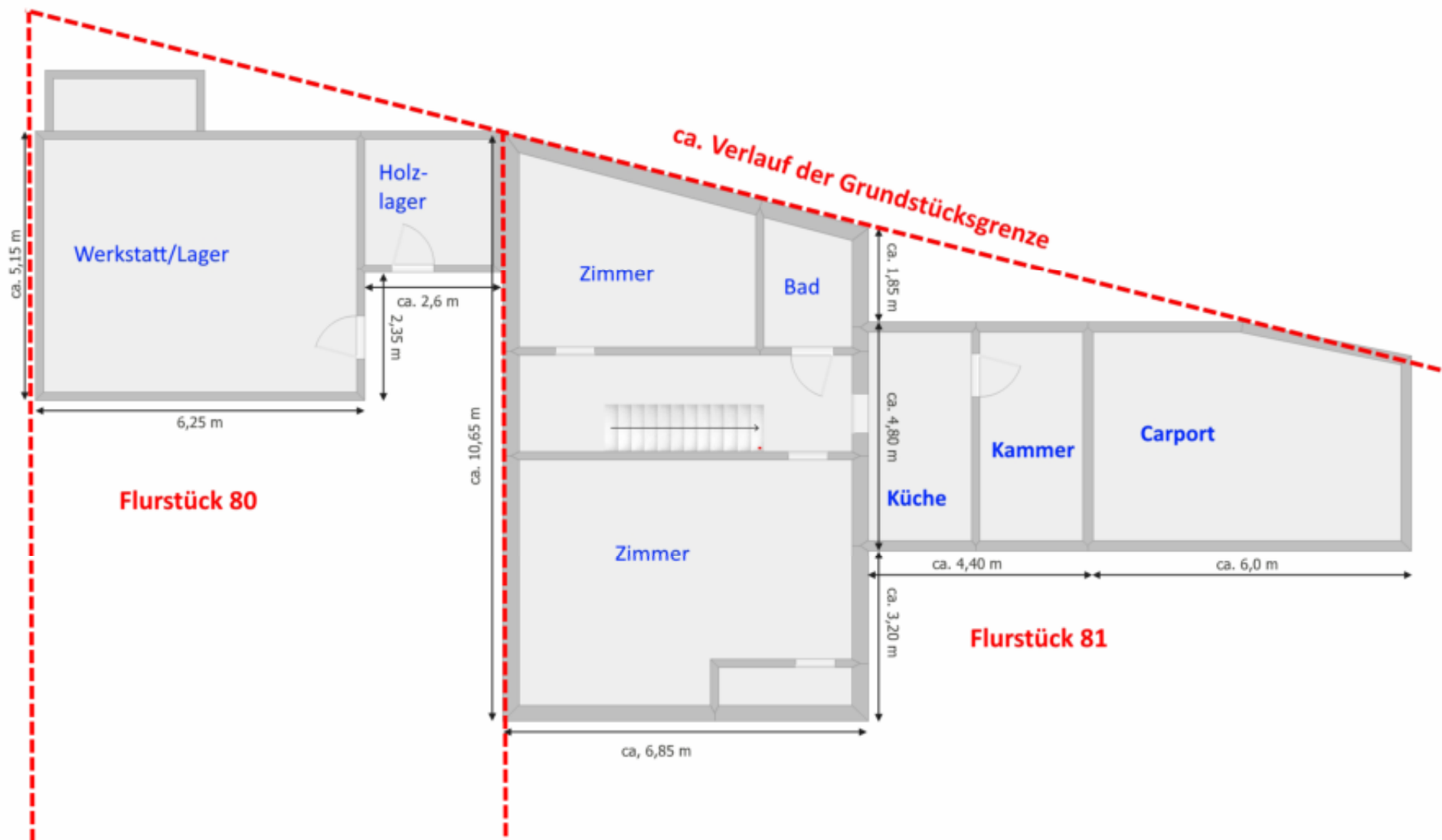
Ungefäher schematischer Grundriss vom Gebäude 2 (EG); erstellt vom Gutachter (Genauigkeit ca. +/- 5%)
