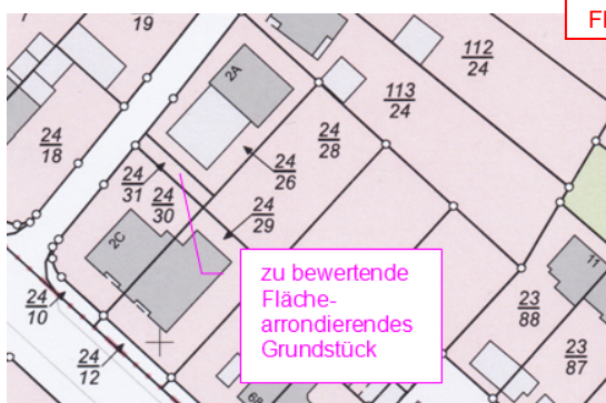
Auszchnitt Flurkarte
