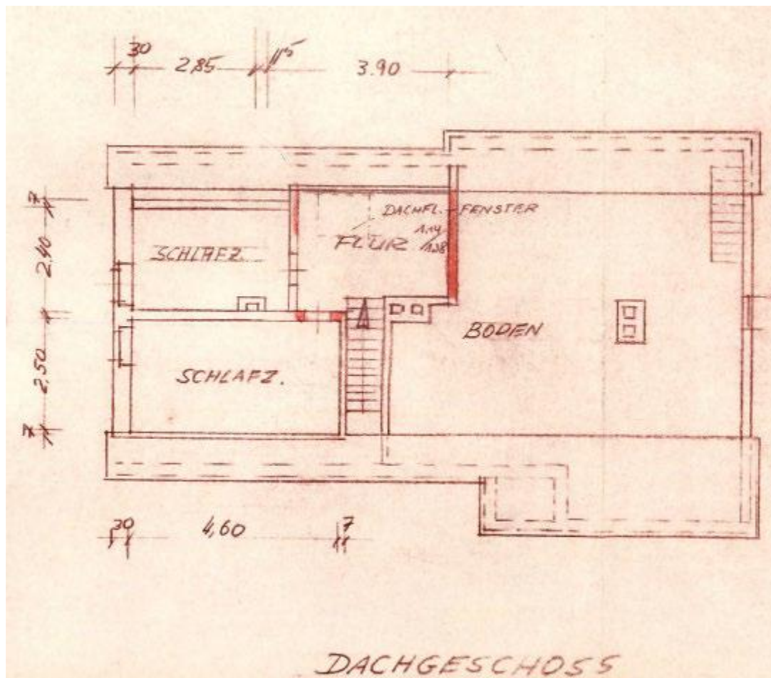
Grundriss Dachgeschoss
